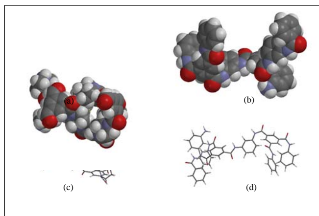
Rajah 14 Model pengisian ruang: (a) PIP-TMC poliamida, (b) BA-TMC poliamida, dan tiub model bagi (c) PIP-TMC poliamida dan (d) BA-TMC poliamida
